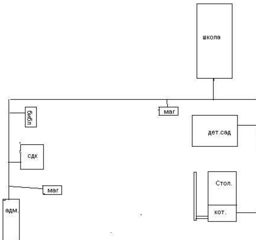
Рис. 2.3.1. Схема тепловой сети котельной с. Маловолчанка
